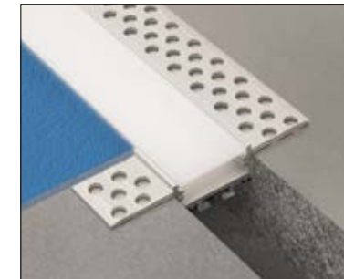
Incasso a raso 359 incasso filomuro F [100-300cm] Cartongesso ESCLUSO
